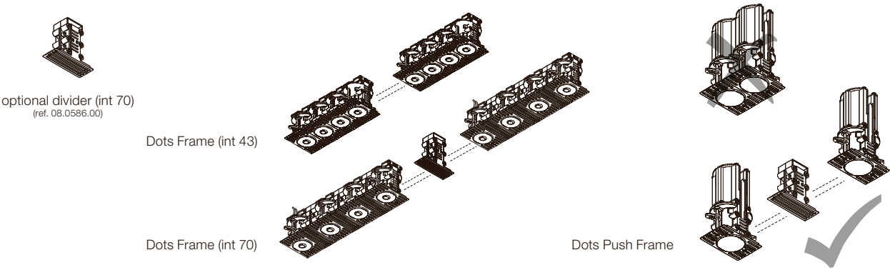
Interconnection information to build a continuous line / Detalle de interconexión para construir una línea continua
