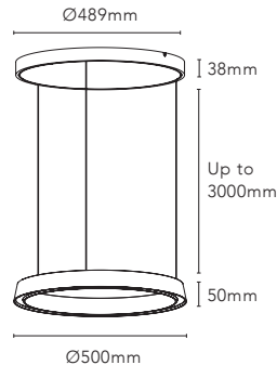
EDGE ROUND Ø500
