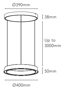
EDGE ROUND Ø400
