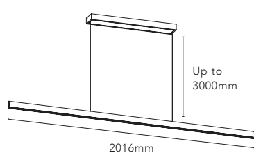
EDGE LINEAR S2000
