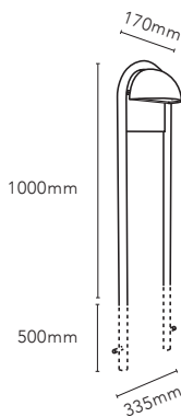
RØRHAT STAND XL
