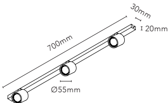
FOCUS MINI L700
