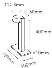
ORBIT GARDEN MINI
